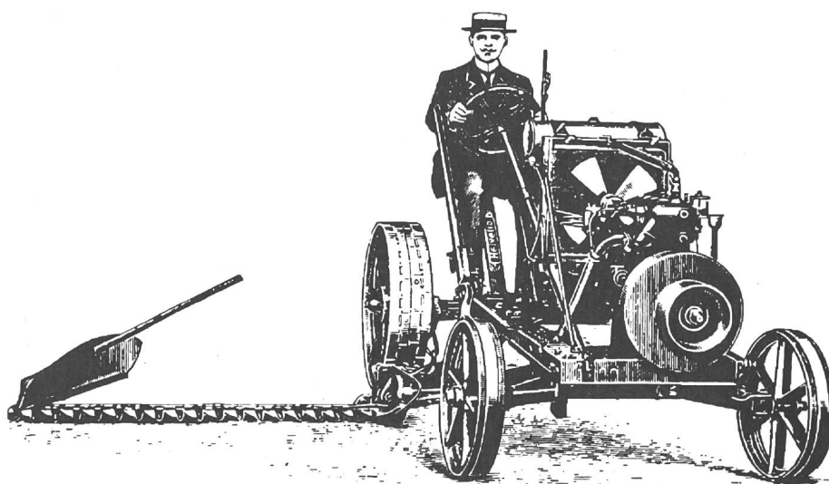
Tracteur-faucheur Helvetia, moteur à essence 6 CV, poids 700 kg, année de construction 1915, fabricant AEBI, Berthoud. Avis de recherche: tout propriétaire d'une quelconque rareté ou de documents techniques, photographies, prospectus est prié de s'annoncer en tenant compte de la liste ci-contre.
