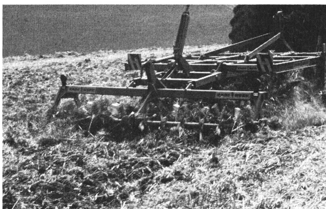
Fig. 4: Les outils suiveurs émiettent et égalisent le sol. Le peigne avec rouleau à lattes (RabR, à droite) le raffermi en plus, contrairement aux bêtes roulantes (RabB, à gauche).
