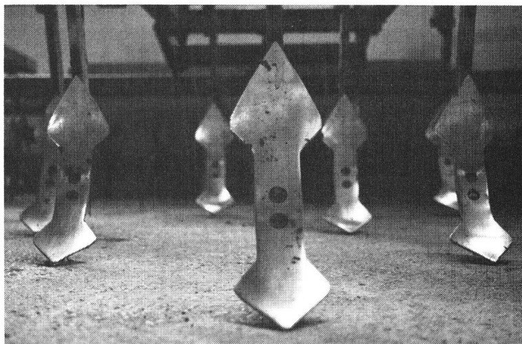
Fig. 8: Contrairement aux socs bombés (Rab0, à droite), les socs à ailettes (Lemk, à gauche) travaillent le sol sur toute la surface. Lors d'un travail plus profond d'environ 15 cm, ils ne font que passer à travers la terre sans la mélanger suffisamment.
