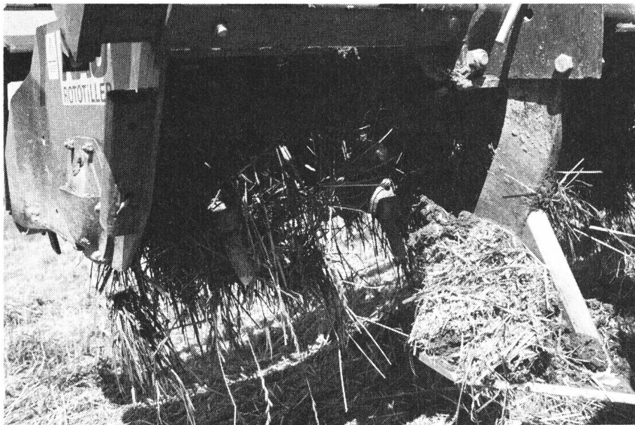
Fig. 19: La rangée de dents avant de la herse rotative à axe horizontal (Rau) réduit l'usure des dents du rotor et permet de maintenir une profondeur de travail constante même à des vitesses d'avancement relativement élevées. En présence de paille hachée, elle risque cependant de se boucher.
