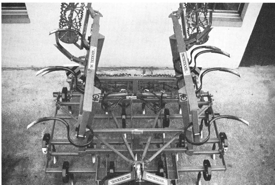
Fig. 10: Pour le transport, le vibroculteur (Koec) est replié verticalement. Le maniement ne pose pas de problèmes.
