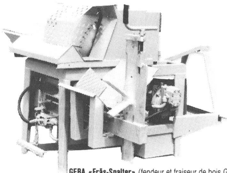
GEBA «Fräs-Spalter» (fendeur et fraiseur de bois GEBA) fraise et fend le bois de chauffage en une seule opération. Type FS-Z pour entraînement de la fusée de l'arbre. Types FS-ZE pour entraînement de la fusée de l'arbre et électromoteur de 9,5 kW à ajouter.
