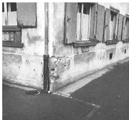
Avant l'application du système Electro-osmose-Assèchement des murs en 1980.
