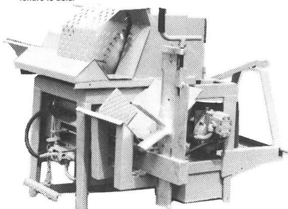
Le scie circulaire-fendeuse à bois GEBA scie et fend le bois de feu en une seule opération. Type FS-Z pour entraînement par prise de force. FS-ZE pour entraînement par prise de force et moteur électrique 7,5 kW. La grande nouveauté!
