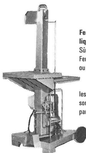
Le scie circulaire-fendeuse à bois GEBA scie et fend le bois de feu en une seule opération. Type FS-Z pour entraînement par prise de force. FS-ZE pour entraînement par prise de force et moteur électrique 7,5 kW. La grande nouveauté!
