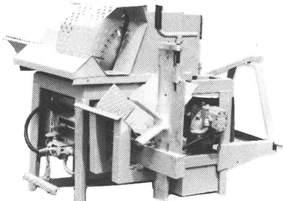
Le scie circulaire-fendeuse à bois GEBA scie et fend le bois de feu en une seule opération. Type FS-Z pour entraînement par prise de force. FS-ZE pour entraînement par prise de force et moteur électrique 7,5 kW. La grande nouveauté!
