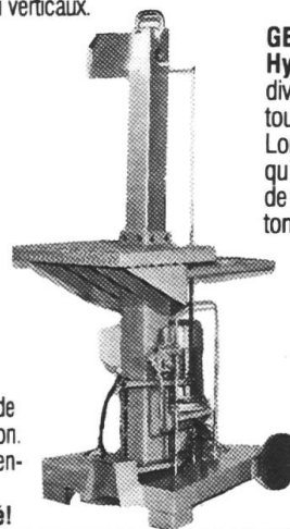
Spaltfix est maintenant encore plus robuste, plus sûre et d'un rendement meilleur. Modèles pour bois, horizontaux ou verticaux.
