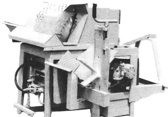
GEBA «Fräs-Spalter» (fendeur et fraiseur de bois GEBA) fraise et fend le bois de chauffage en une seule opération. Type FS-Z pour entraînement de la fusée de l'arbre. Type FS-ZE pour entraînement de la fusée de l'arbre et électromoteur de 9,5 kW à ajouter. La grande nouveauté!
