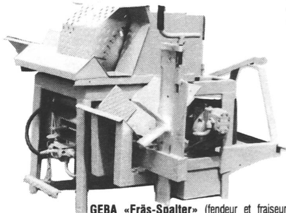
GEBA «Fräs-Spalter» (fendeur et fraiseur de bois GEBA) fraise et fend le bois de chauffage en une seule opération. Type FS-Z pour entraînement de la fusée de l'arbre. Type FS-ZE pour entraînement de la fusée de l'arbre et électromoteur de 9,5 kW à ajouter.
