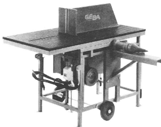
GEBA 85 , la nouvelle fraiseuse standard aménageable. Robuste, solide, grande table, dispositif pour fentes à ajouter.
