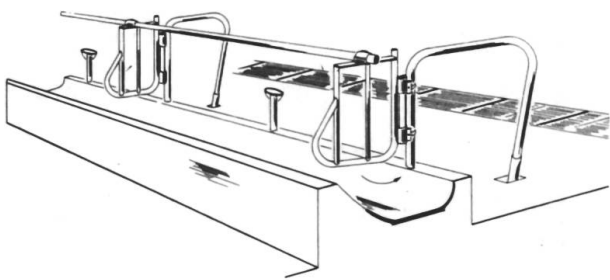
Système d'attache STALLAG "Enorm-Plus" modèle "E"
