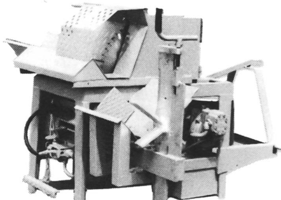
La scie circulaire-fenduse à bois GEBA scie et fend le bois de feu en une seule opération. Type FS-Z pour entraînement par prise de force, FS-ZE pour entraînement par prise de force et moteur électrique 7,5 kW. La grande nouveauté !
