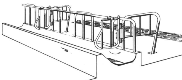
Système d'attache STALLAG "Titlis" modèle "FS" avec étrier ouvrant pivotant OVF no 14257
