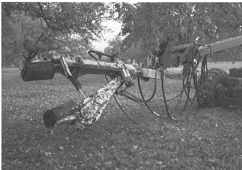
La pince saisit l'arbre et le secoue un instant, pendant lequel les fruits mûrs tombent à terre.
