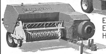
RAMASSEUSE-PRESSE SGORBATI
