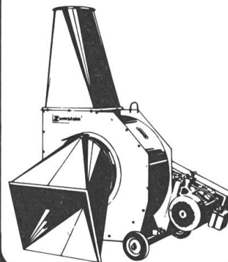
Installation de séchage du foin, système radial. La série encore améliorée des ventilateurs radiaux à haut degré d'efficacité (4-25 CV). Testés par la FAT. Commande automatique.
