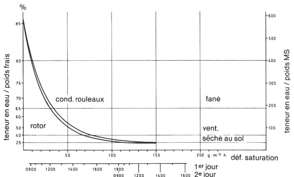
Fig. 5: Les conditionneuses à rouleaux suivent de près les conditionneuses à rotor pour ce qui est de l'accélération de séchage.
