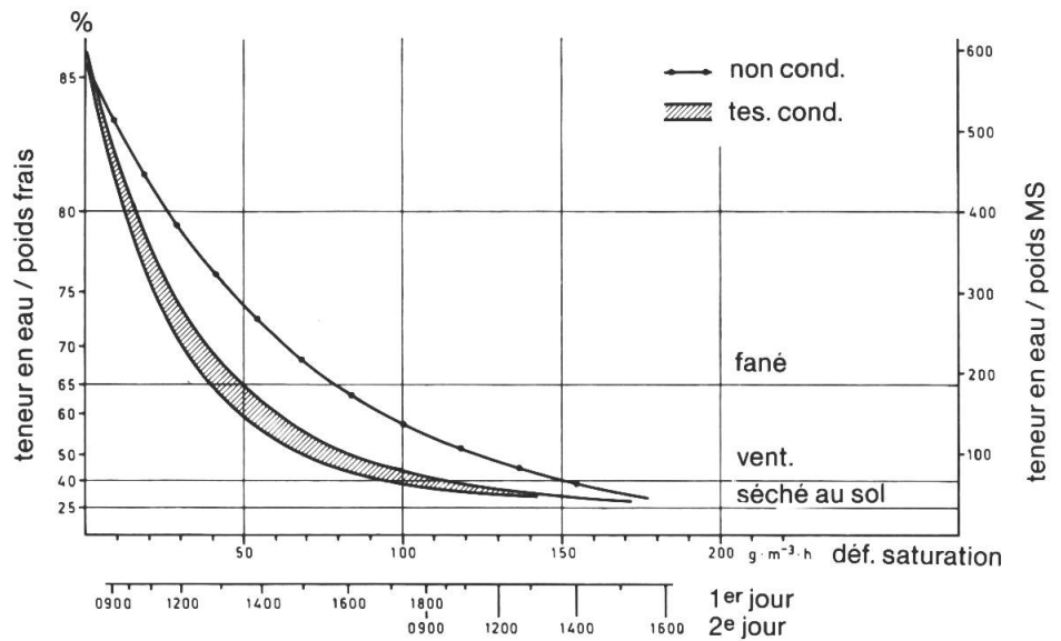
Fig. 4: Courbes de dessiccation obtenues avec les machines testées, comparativement à une faucheuse sans conditionneuse.
