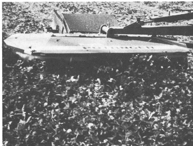
Fig. 3: Un fourrage riche en feuille exige un réglage particulièrement précis de la machine.
