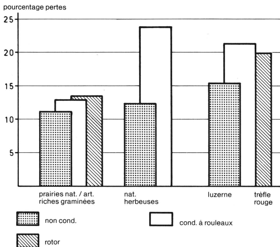
Fig. 6: Pertes de matière sèche, en % de la récolte fraîche, pour divers types de récoltes.
