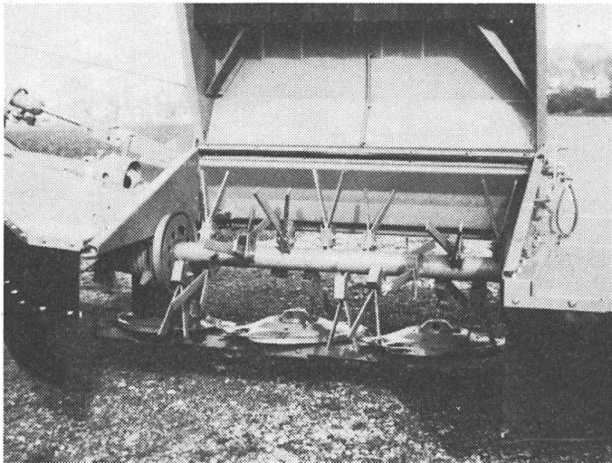
Fig. 7: De bonnes possibilités d'accès facilitent grandement le nettoyage.
