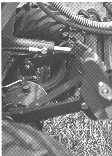
Un nouveau coupleur rapide relie l'essieu avant de la motofaucheuse avec les outils portés.
