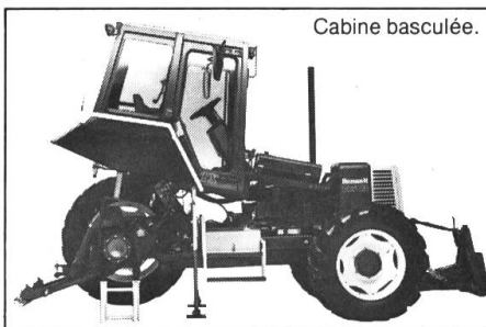
Cabine basculée.
