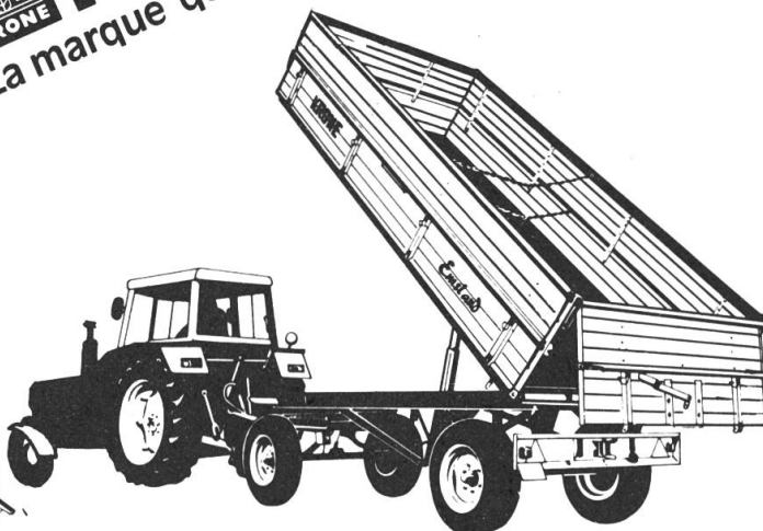
Remorques basculantes 3-côtés, à 2 essieux, avec ridelles en Alu éloxé.
