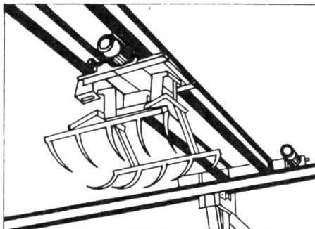
Fig. 1: Autochargeuse surbaissée TL-200.
