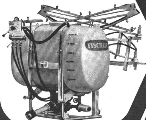
Pulvérisateur porté AGRIFIX
