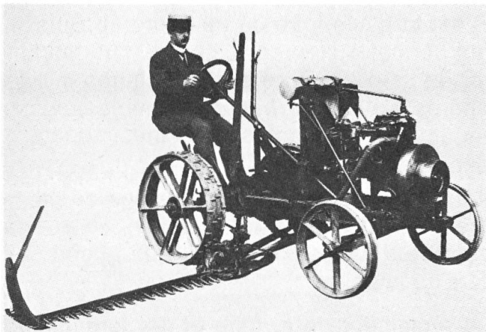
Faucheuse automobile «Helvetia» Photo: Aebi & Cie, Berthoud (1915)
