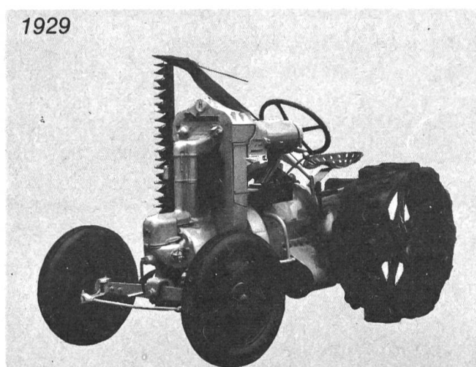
Tracteur Hürlimann (1929) 1er modèle à 1 cyl. Moteur à essence Bernard. Fabriquait H. Hürlimann, Wil. Nous publions ces 2 photos avec la gracieuse collaboration de H. Gerber-Crot, 4104 Oberwil BL.
