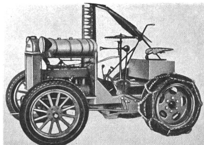
Tracteur Bühler (1929), 1er modèle avec moteur Ford T, 4 cyl. (White Sirit), fabriqué par F. Bühler, Frauenfeld. (Photo H. Beglinger †).
