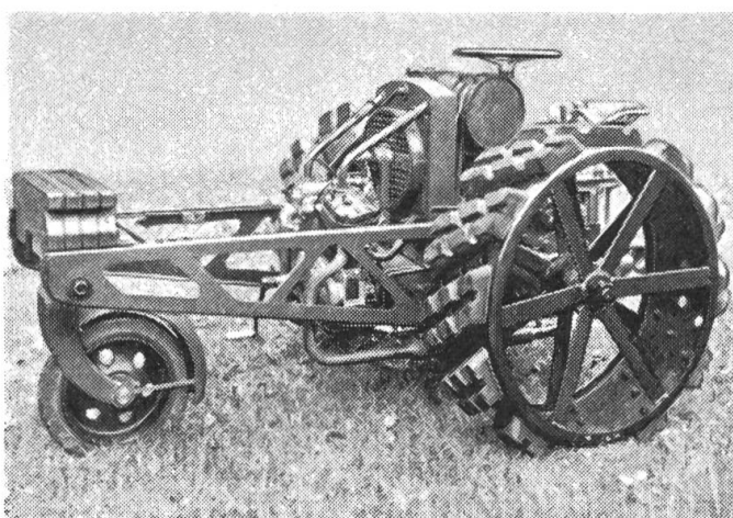
Tracteur Mafag (1929) qui fut un Universal amélioré. Construit par la Fabr. de machines Brougg. (Photo H. Beglinger †).
