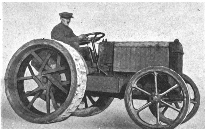
Tracteur Austin (1920), importé de France par la maison Blatter à Zurich, moteur à essence, 4 cyl. (Photo H. Beglinger †).
