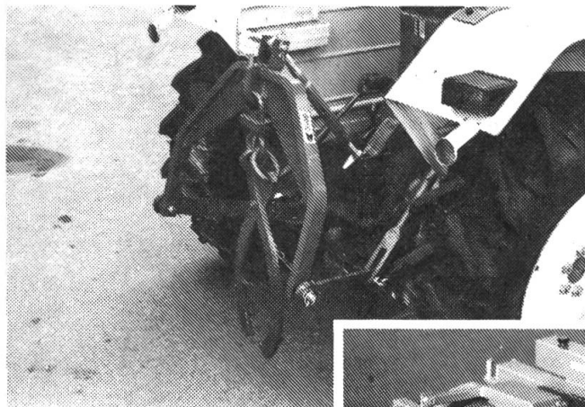
Joug d'attelage avec tenailles pour débardage de troncs d'arbres
