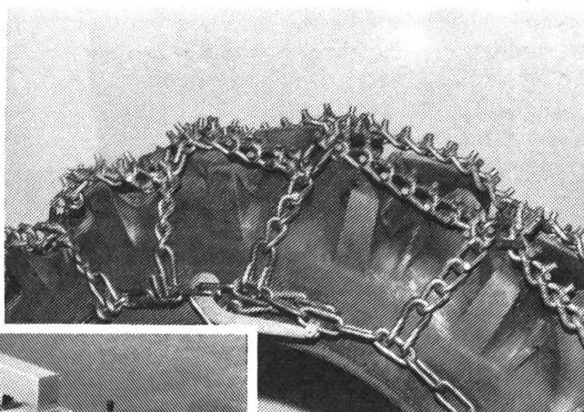
Chaînes antidérapantes Trygg pour exploitations forestières et parcs à machines communaux. Minimum d'usure, bonne garde au sol; ménage les revêtements en asphalte.
