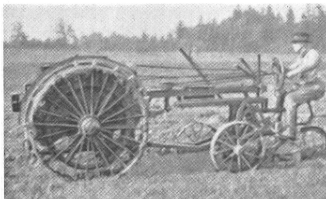
Tracteur Universal-Moline (1917), importé par la maison U. Ammann, Langenthal BE, mot. à essence de 12 CV, 2 cyl. Transformable p. les transports sur route.
