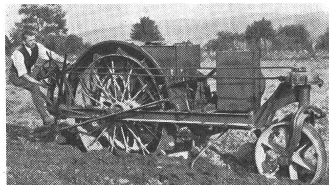
Tracteur Case (1918), des E.U., mot. de 9/18 CV à essence/pétrole. Propriétaire: Commission des cultures de Kloten. A été utilisé sur la place d'exercice de Kloten.
