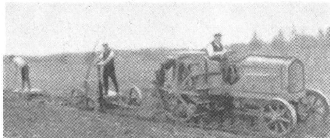
Motocharrue Avance (1917), importée de Suède par la fabrique Bucher-Manz, Niederweningen ZH. Moteur monocyl. à huile lourde, charrue à 2 ou 3 socs.
