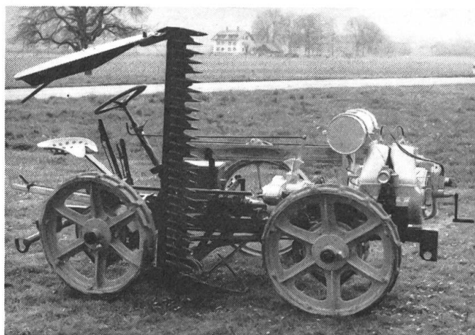
Fig. 2: Faucheuse automotrice Aebi à trois roues (modèle 1927). Reconstituée par les agromécaniciens de l'Ecole professionnelle de Liestal.
