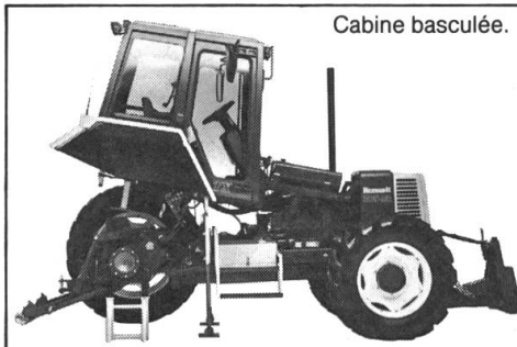
Cabine basculée.
