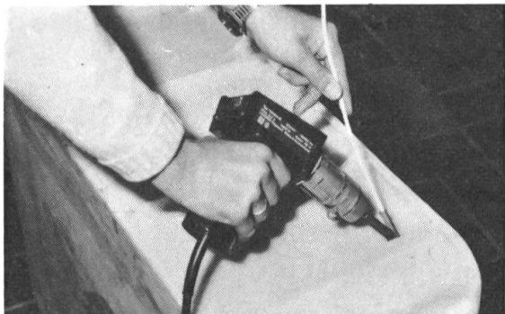
Le LEISTER pendant la réparation d'un container en polyaéthylène.
