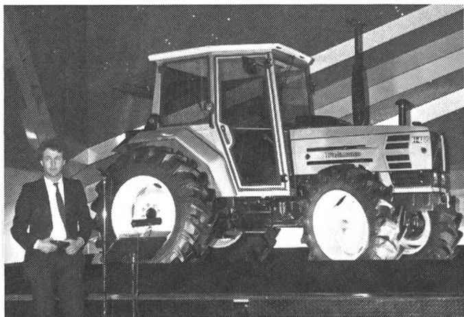
Fig. 3: Monsieur Max Hürlimann présente le modèle 466 sur la scène de la salle de démonstration. Moteur de 65 CV (48 kW), boîte de vitesses standard 24 x 12, 4 vitesses, engrenage à demi-vitesse et renversement synchronisés. Une version de transport de ce même modèle est également livrable.
