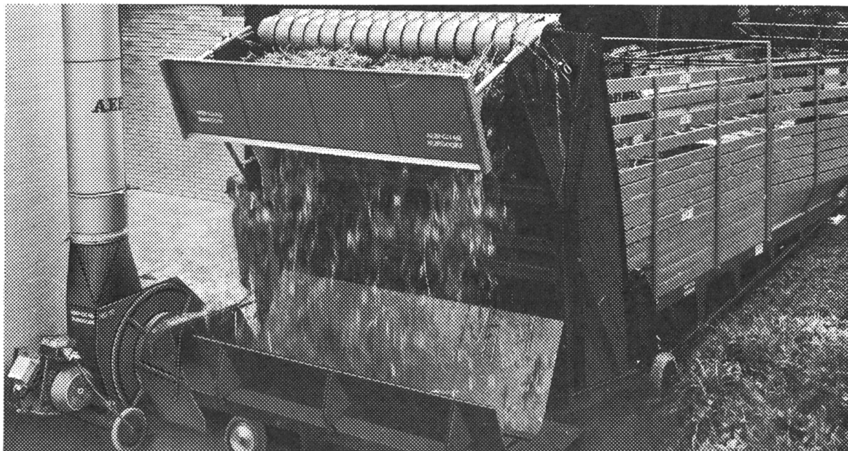
4 souffleurs à aspiration HG 0, HG 1, HG 8 et HG 9 pour fourrage sec et préfané
