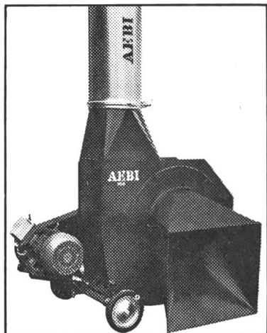
4 souffleurs à aspiration HG 0, HG 1, HG 8 et HG 9 pour fourrage sec et préfané
