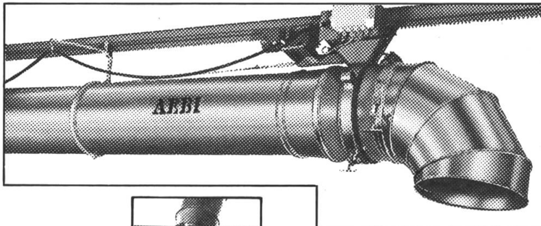
Distributeur télescopique pour grandes surfaces, dirigeable à partir du sol, avec dispositif d'épandage en arrière, crémaillère sans poutre en bois
