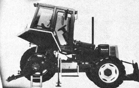
Cabine basculée.
