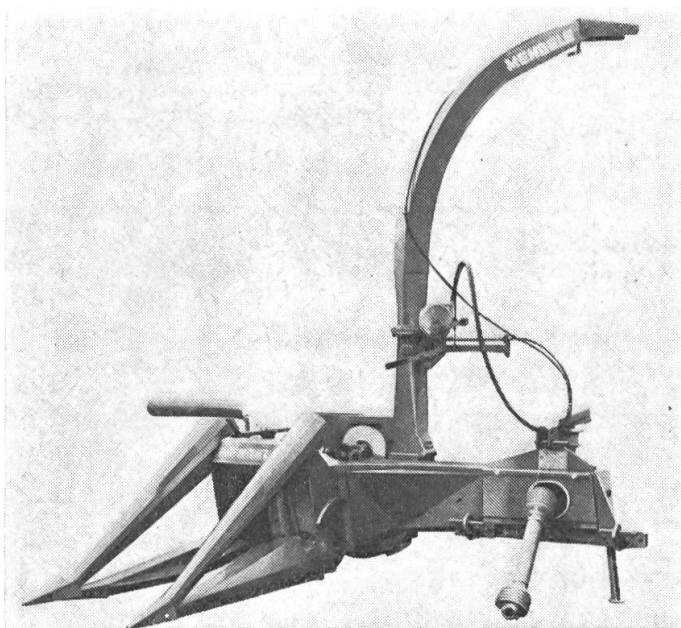
Fig. 1: Récolteuse-hacheuse à maïs portée MB 200/280.
