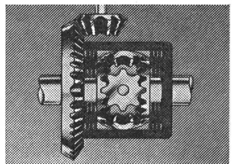
Notre transmission entièrement intégrée tire directement sa puissance de la transmission centrale. Des disques placés sur les planétaires du différentiel, limitent automatiquement tout patinage dès qu'une roue commence à perdre de l'adhérence.
