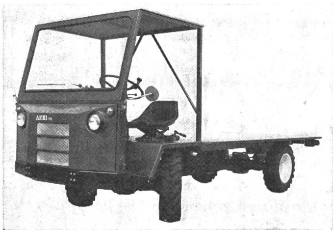
Fig. 1: Le nouveau char automoteur AEBI TP 25.
