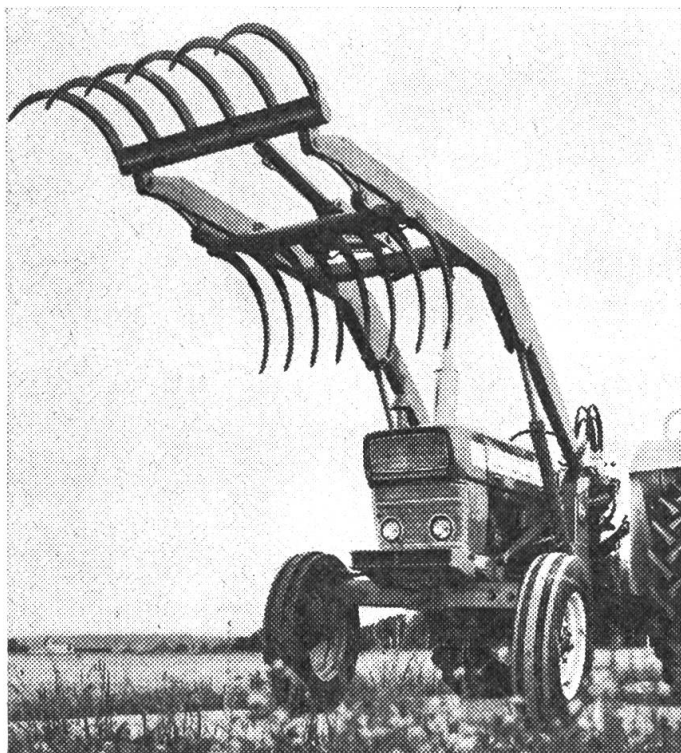
CHARGEUR FRONTAL «GLOUTON» Brevet suisse et étranger
