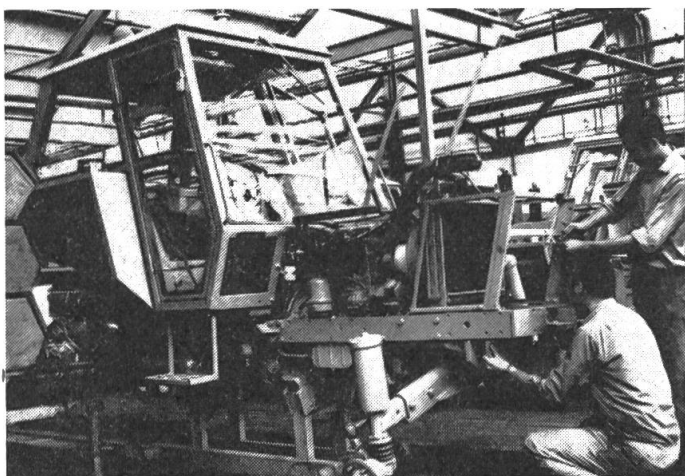
Fig. 1: Une des chaînes de montage des usines Zetor en Tchécoslovaquie.
