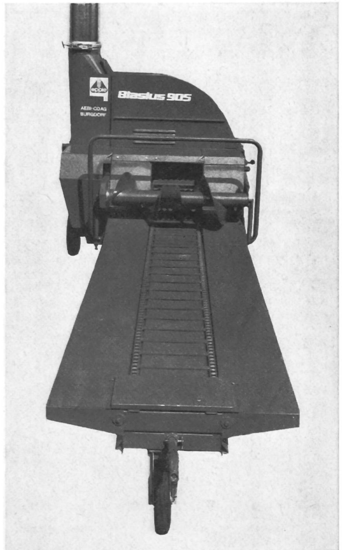
Hacheuse-ensileuse Blasius 905
