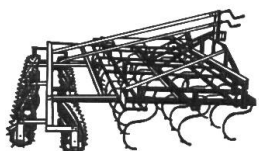
Herses avec dents à ressort réglables MÜLLER avec émotteuses à 1 ou 2 rouleaux
