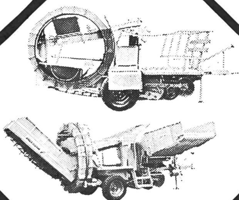
Arracheuses de pommes de terre Wisent, cau- sant peu de dégâts!
