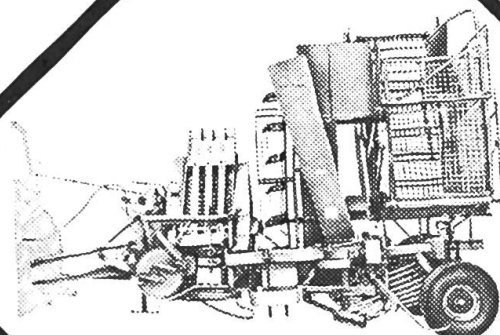
Arracheuses de betteraves Ratio- nal, la machine qui écono- mise la main-d'œuvre chère!
