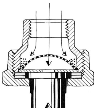
Buse de précision 110° avec filtre auto-nettoyant.
