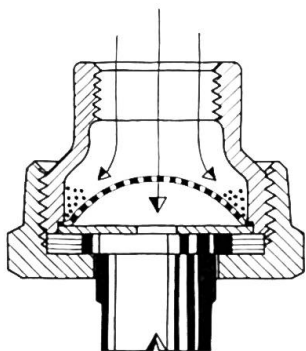
Buse de précision 110° avec filtre auto-nettoyant.
