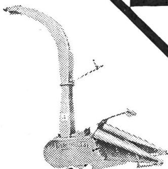
Ensileuse de maïs Hagedorn, tambour rotatif à grande vitesse avec 9 cou- teaux, longueur de coupe 4,5 à 6 mm, capacité de 25 à 30 t/h, vitesse de travail 5 à 8 km/h puissance requise 30 à 60 CV
