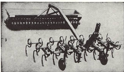
Ensemble porte outil-Vibroculteur-Cultipacker
