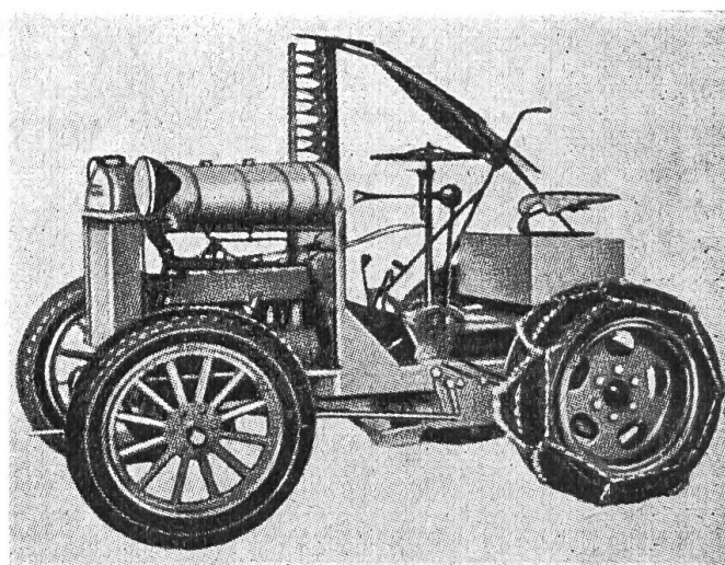
Tracteur Mafag qui fut un Universal amélioré. Construit par la Fabrique de machines de Brougg.
