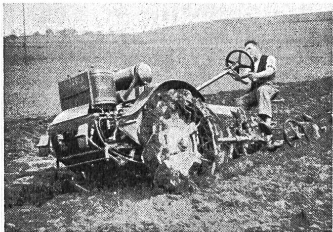
Tracteur Agro importé de France par la Centrale de machines d'Yverdon.
