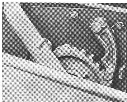
Système de relevage du picup breveté.
