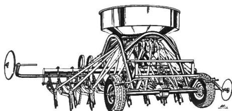
Semoirs de céréales conventionnels HASSIA et centrifuges KVERNELANDS
