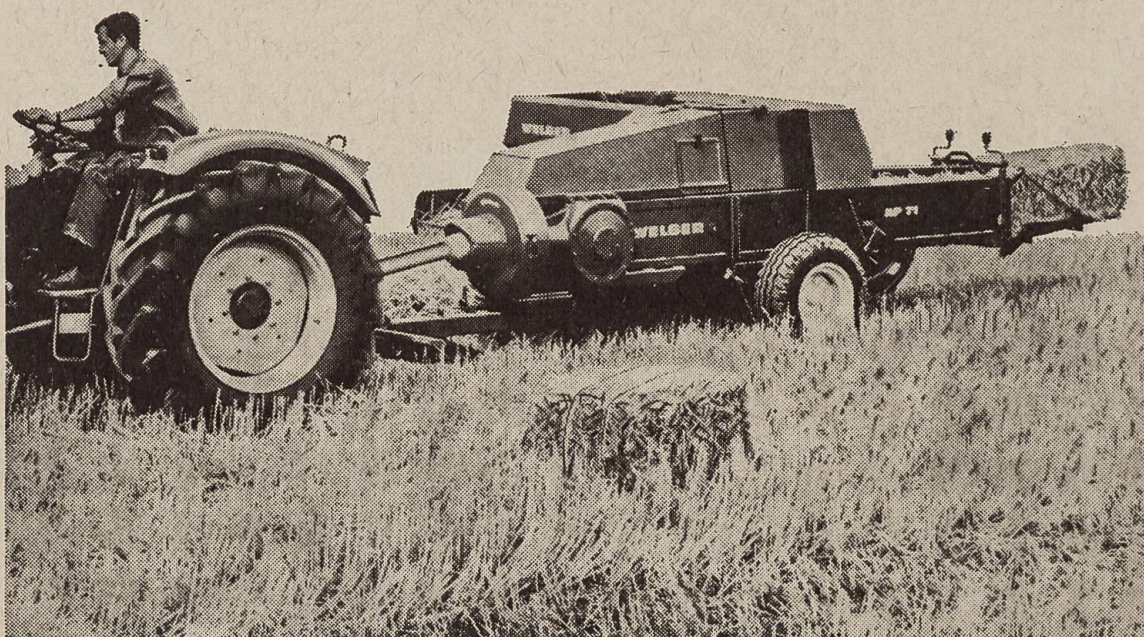
Système de relevage du picup breveté.
