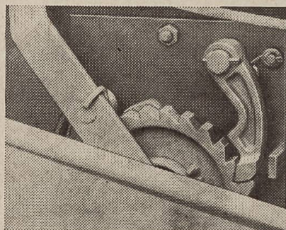
Système de relevage du picup breveté.
