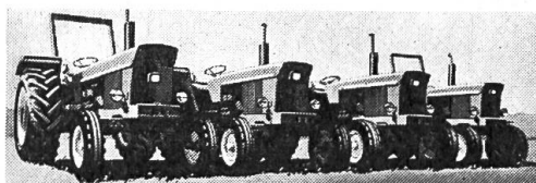
Tracteurs John Deere 1630 (59 CV), 2030 (71 CV), 2130 (79 CV), 3130 (97 CV).
