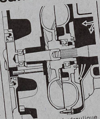
Embrayage turbohydraulique
