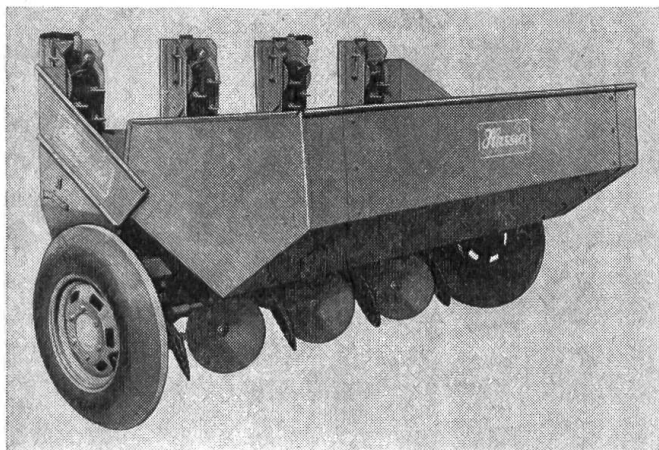
Aspect de la nouvelle planteuse de pommes de terre Hassia, modèle GLB, avec chaînes de distribution à double rangée de godets et grande auge d'approvisionnement basculable.
