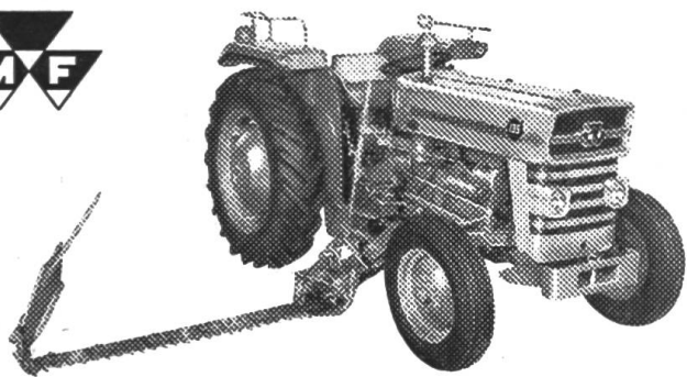
La nouvelle faucheuse portée entre roues MF 173 à relevage hydraulique, équipée avec barre « Rasant » 150 cm.
