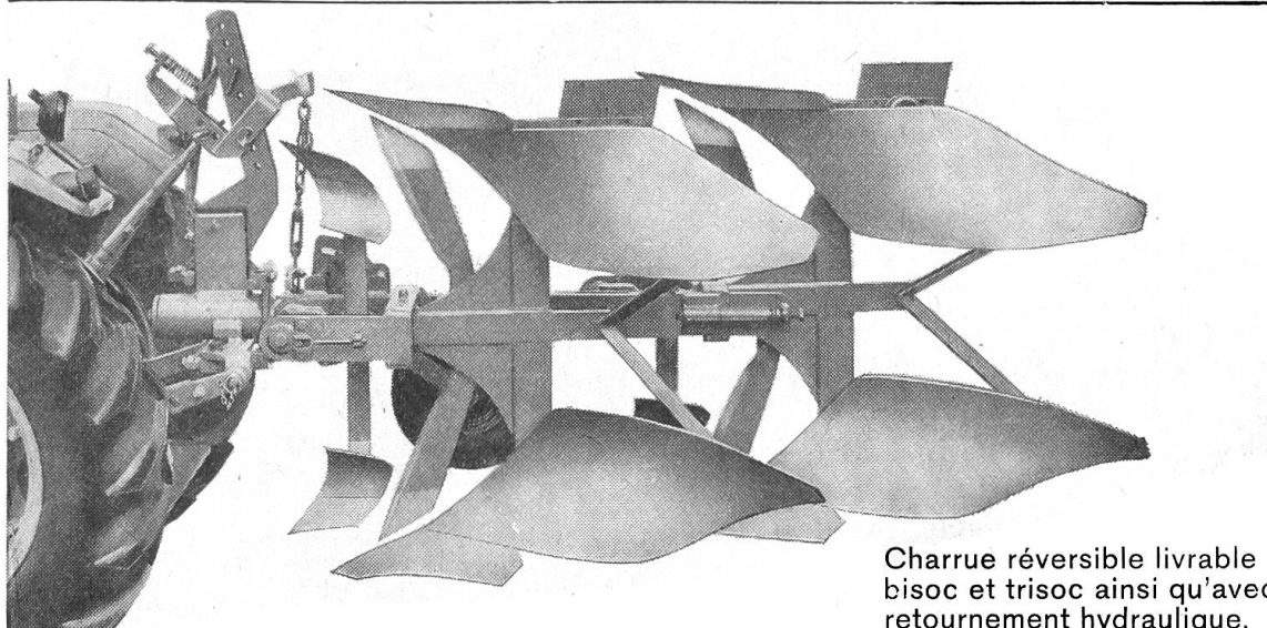
Charrue réversible à \frac{1}{4} de tour monosoc. La charrue idéale pour chaque entreprise.
